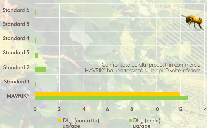
Confronto della DL 50 * di diverse sostanze attive su api (Fonte: Pesticide Properties Database)
